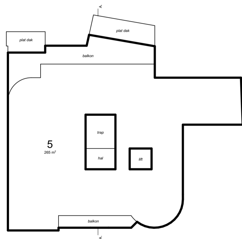
1e VERDIEPING schaal 1:200
